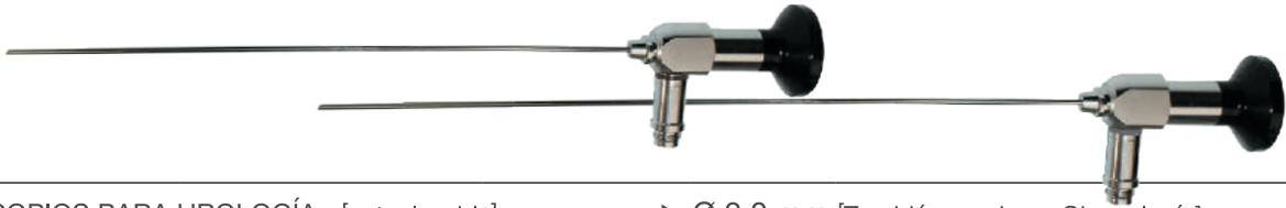
TELESCOPIOS PARA UROLOGÍA [autoclavable] ▶ Ø 2,0 mm [También usado en Ginecología]
